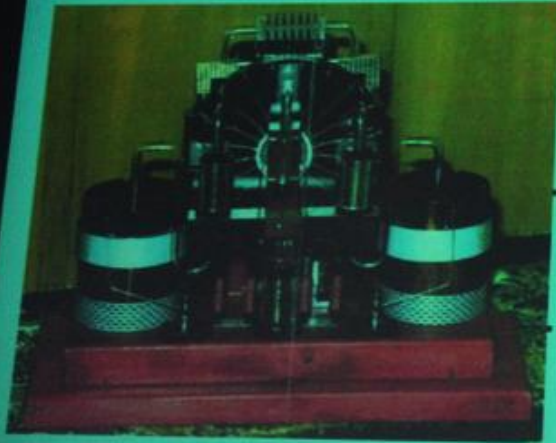
300-Watt-Maschine mit Magneten
