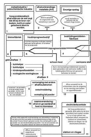
Blokdiagram: van hoog problematisch afval tot groene stroom (klik voor vergroting)
